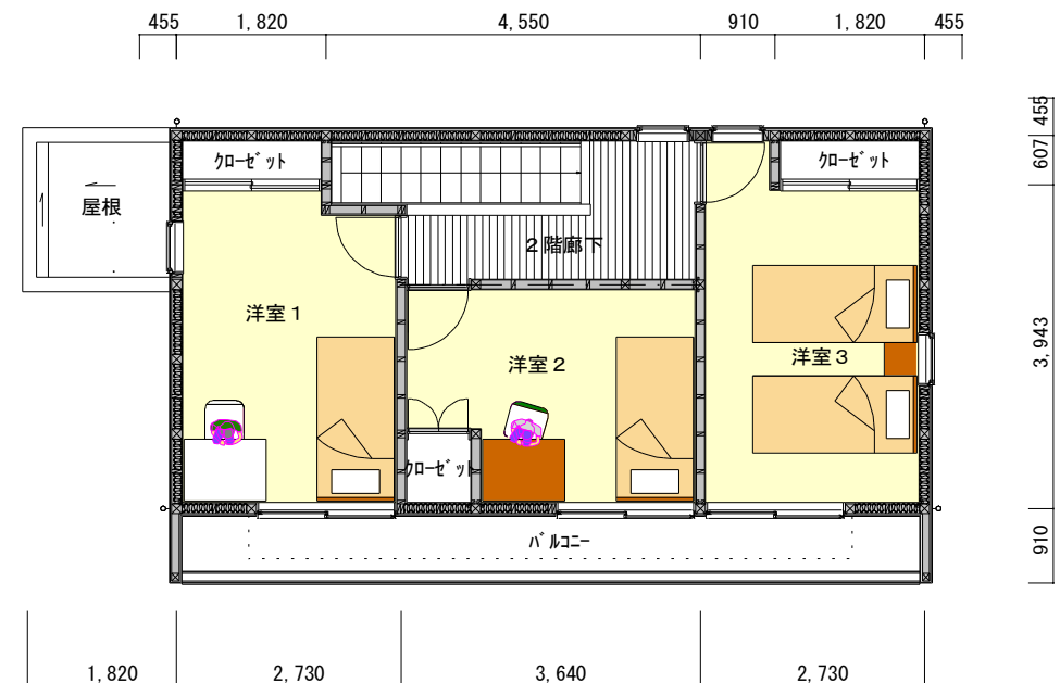
◇ 2階平面図
