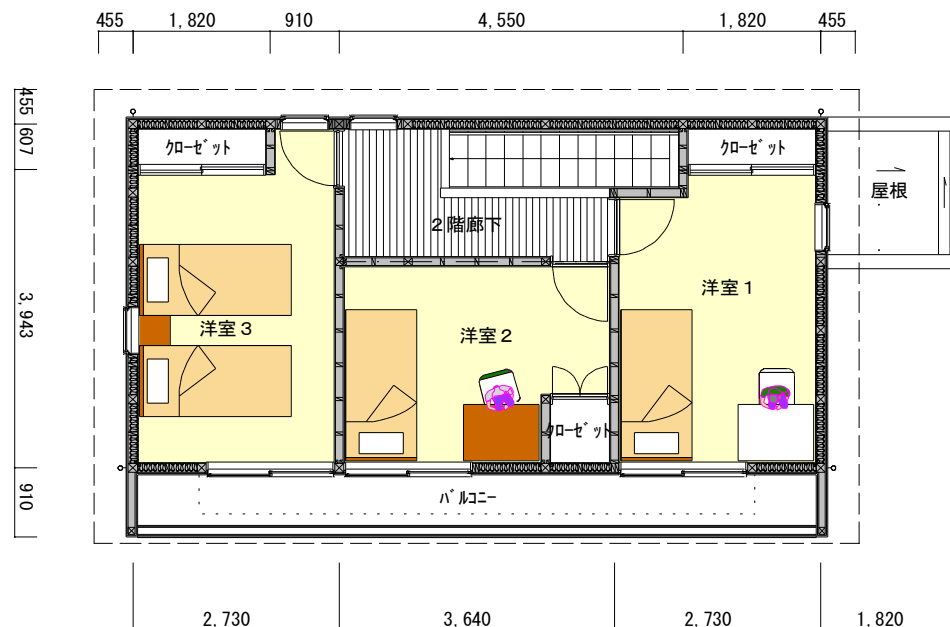
◇ 2階平面図
